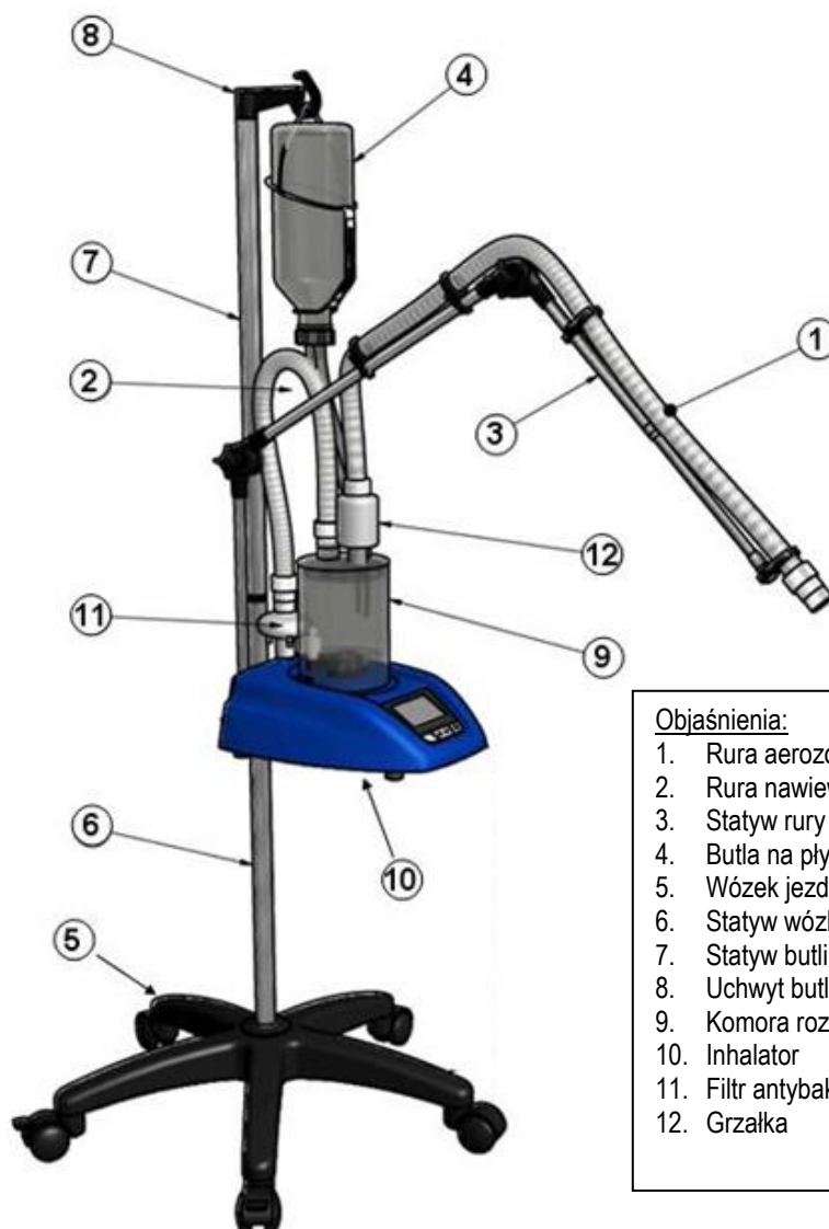
Rys.1: Inhalator ultradźwiękowy „NEB TIME UN-600A” – schemat zestawieniowy.
